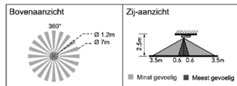
Fig 4: Detectieveld
